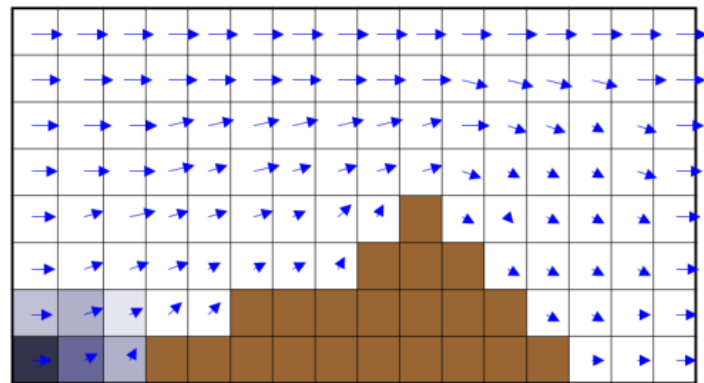
図4 数値計算のイメージ
