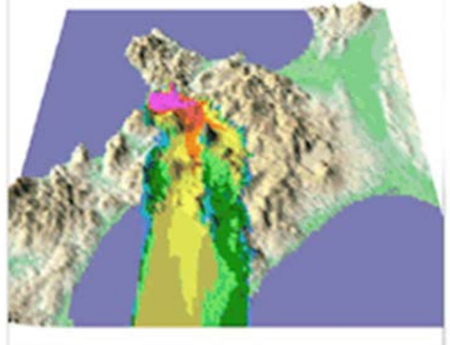
図13 3次元数値計算モデルによる結果
