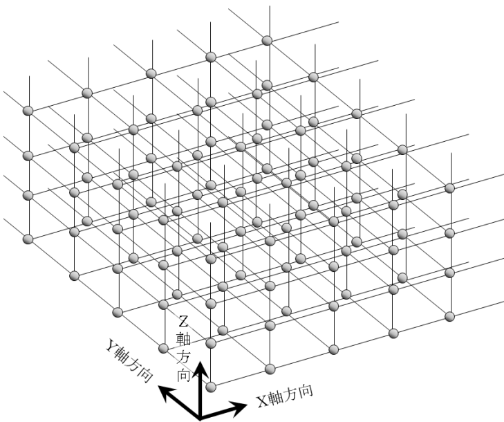
図11 3次元流体計算における計算結果を格納するグリッドイメージ図
