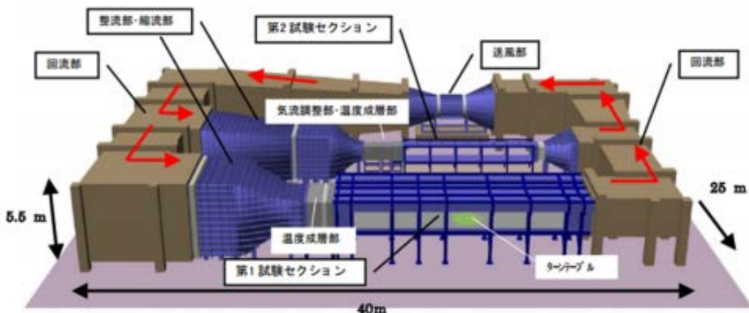
図1 コンピュータ・シミュレーションモデルの精度検証に用いた風洞実験設備
