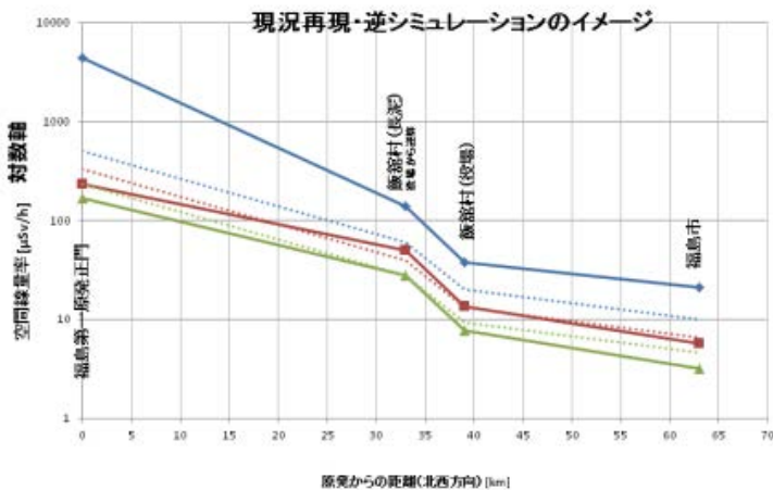
図5 逆シミュレーションデータの例
