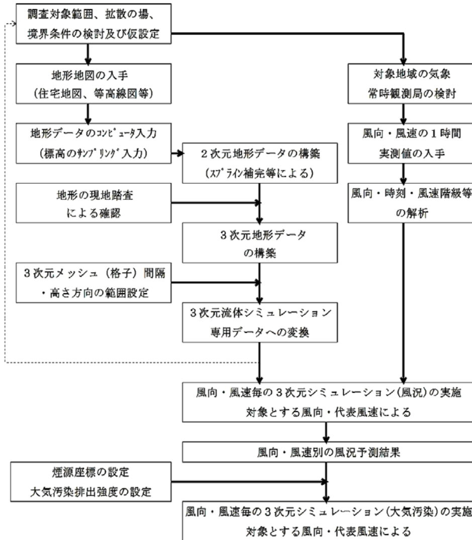
図2 地形を考慮した3次元流体シミュレーションの流れ
